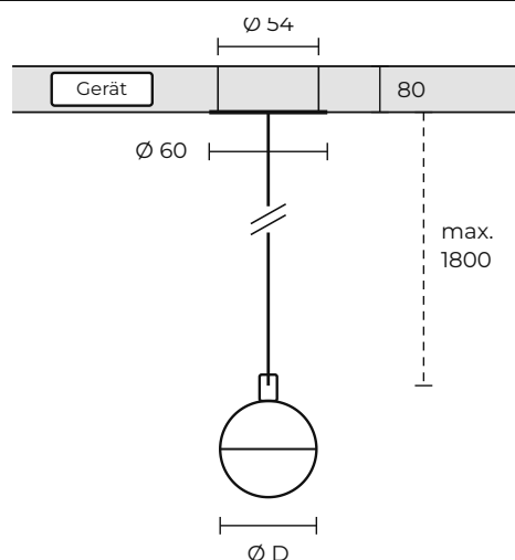
Halbeingelassen – Rosette Ø 60 mm, Einbautiefe 80 mm, Deckenausschnitt Ø 54 mm, Betriebsgerät oberhalb der Decke. D = 60, 90 oder 150 mm. Angaben in mm.
