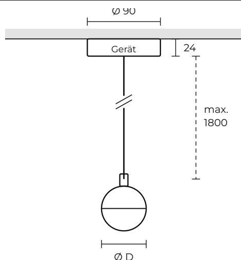
Aufbau – Baldachin Ø 90 x 24 mm mit integriertem Betriebsgerät. D = 60, 90 oder 150 mm. Angaben in mm.
