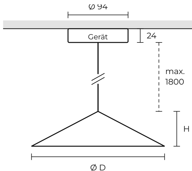
Aufbau – Baldachin Ø 94 x 24 mm mit integriertem Betriebsgerät. D = 265, 327 oder 421 mm, H = 70, 90 oder 120 mm. Angaben in mm.
