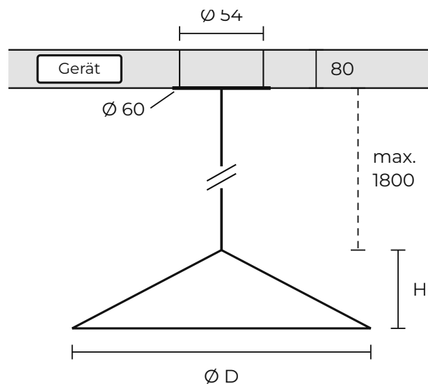
Halbeingelassen – Rosette Ø 60 mm, Einbautiefe 80 mm, Deckenausschnitt Ø 54 mm, Betriebsgerät über der Decke. D und H wie nebenan. Angaben in mm.
