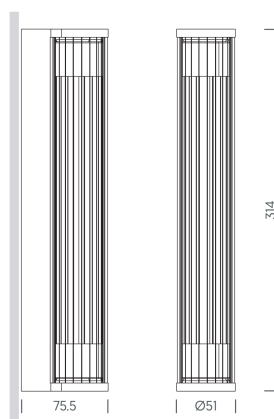
Ansicht und Seitenansicht, Masse in mm
