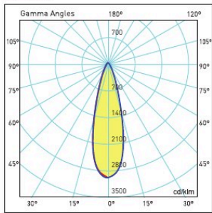
30°Lens
