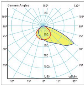
Asymmetric / Asimetrik
