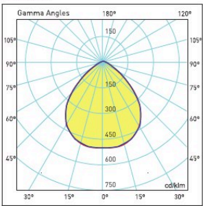
90°Lens
