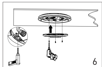
Verwenden Sie einen elektrischen Bohrer, um gemäß den auf der Deckenbasisplatte vorgesehenen Löchern 3 Löcher (Ø2,7 mm) zu bohren. Befestigen Sie dann das Modul mit 3 Schrauben (PA3*10).
