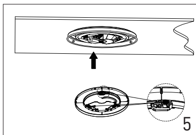
Befestigen Sie das Modul magnetisch an der Deckenbasisplatte (Die Deckenbasisplatte muss aus Metallmaterial bestehen; falls nicht, verwenden Sie Schrauben, um es zu befestigen).
