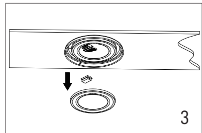
Entfernen Sie die alte Lichtquelle und reinigen Sie die Leuchte vor dem Einbau der Umrüstleuchte.
