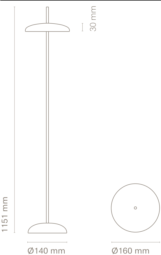
Höhe 1151 mm, Schirm Ø160 mm, Fuss Ø140 mm, Schirmhöhe 30 mm. Masse in mm.
